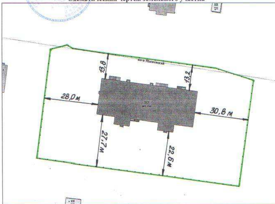
Схематический чертеж земельного участка
